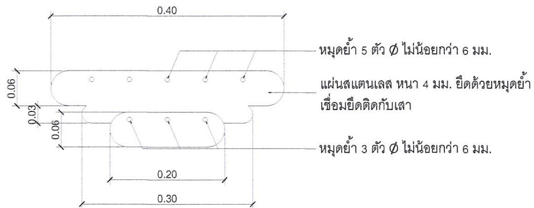
แบบขยาย ① มาตราส่วน 1:25
