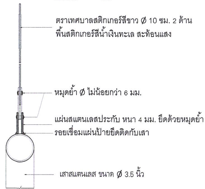
รูปด้านหลัง มาตราส่วน 1:25
